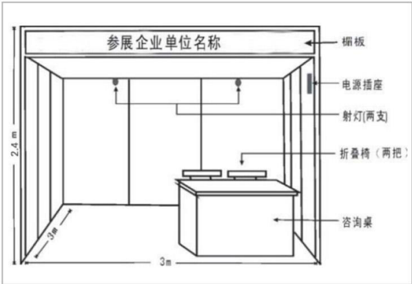
标准展位示意图
